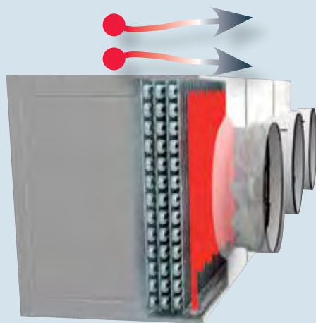
Abtauen ohne FabricAir® DefrostDuct™
