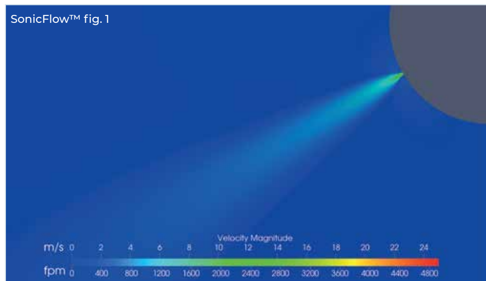
Luftaustritt durch SonicFlow™ - bei 120 Pa
